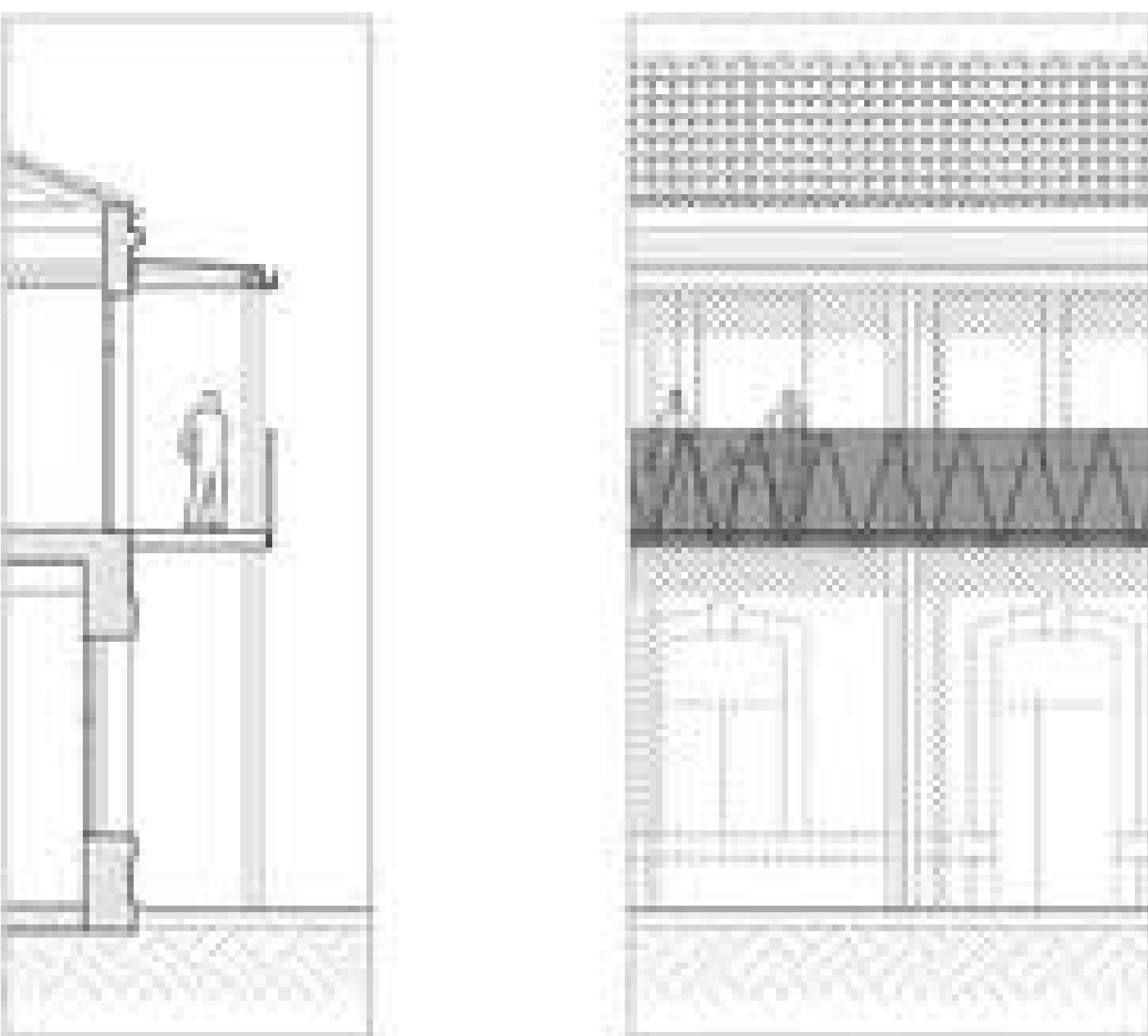
Elevé de principe
